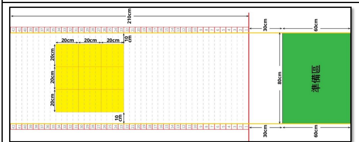
圖 9-3 競賽用場地尺寸標示
